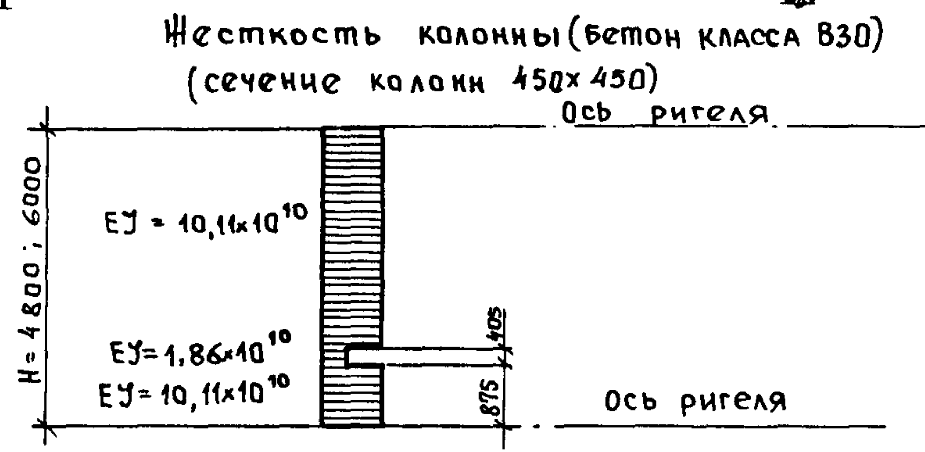
Чертеж №4
