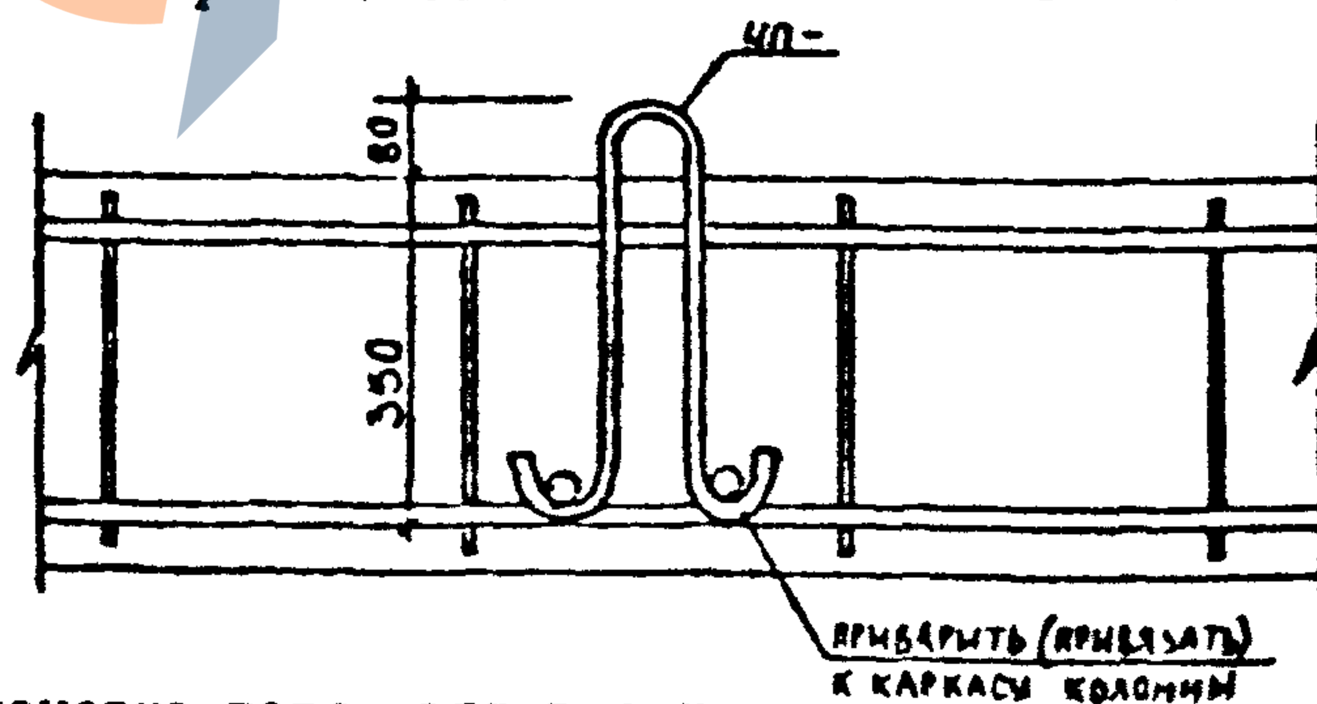
Схема I. Установка петли для выемки колонны из формы и транспортирования Лх. 32830 л. 35
