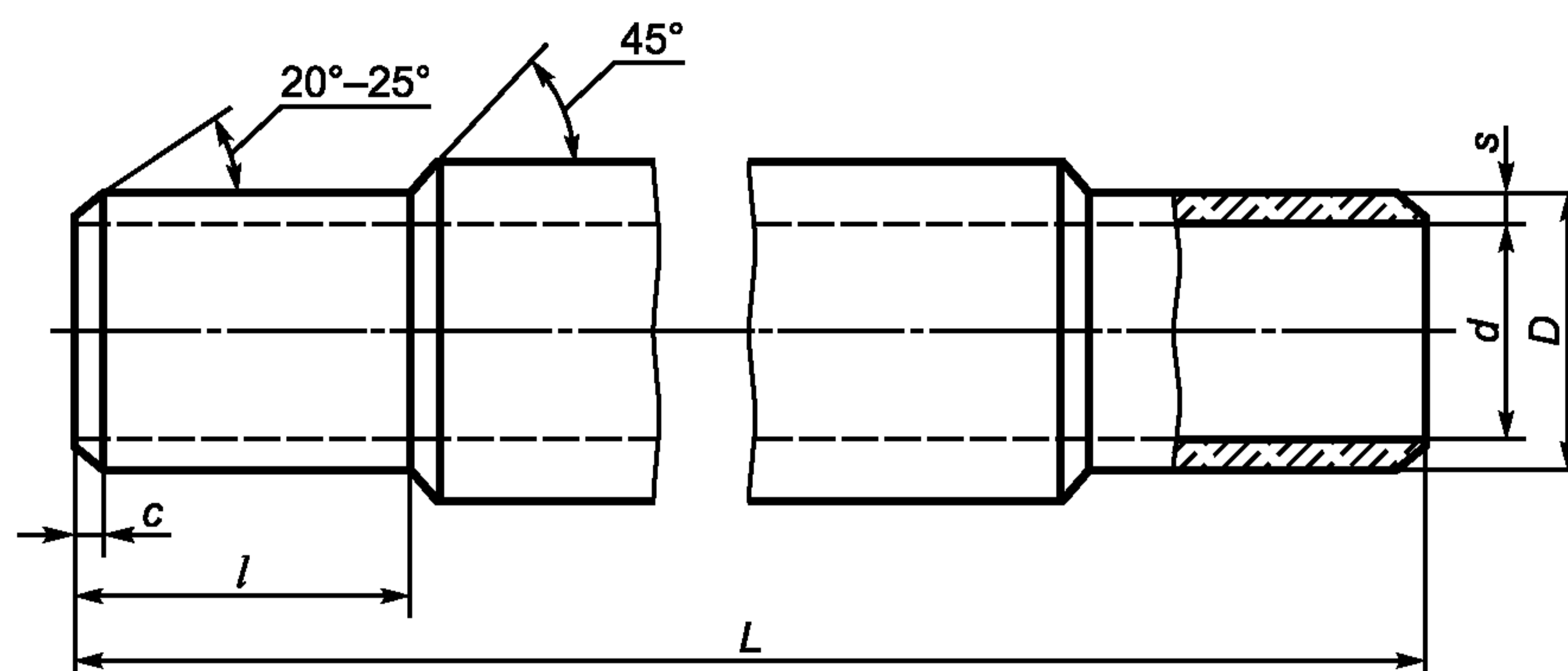
Рисунок 3 — Напорная труба
