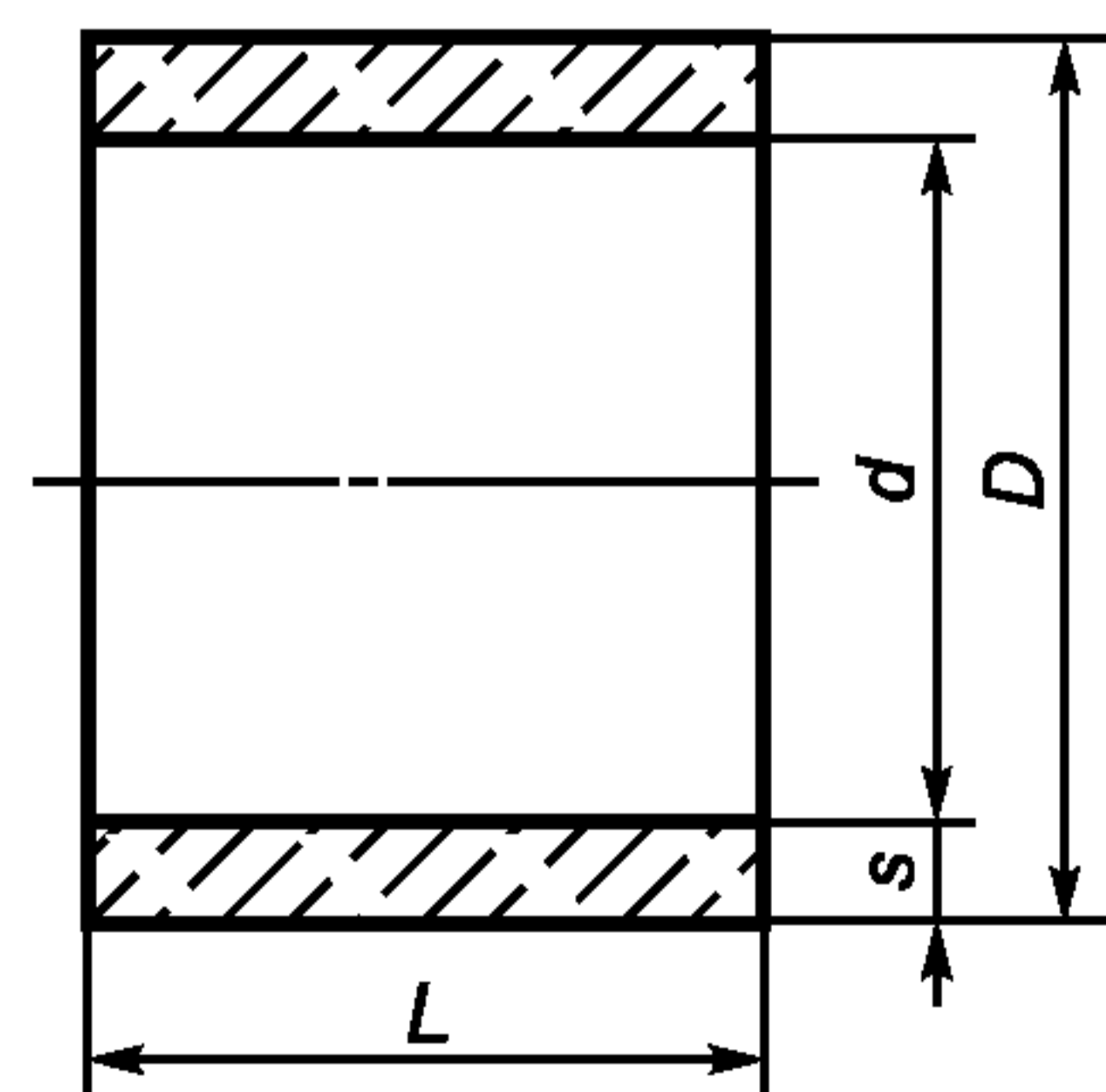
Рисунок 2 — Безнапорная муфта
