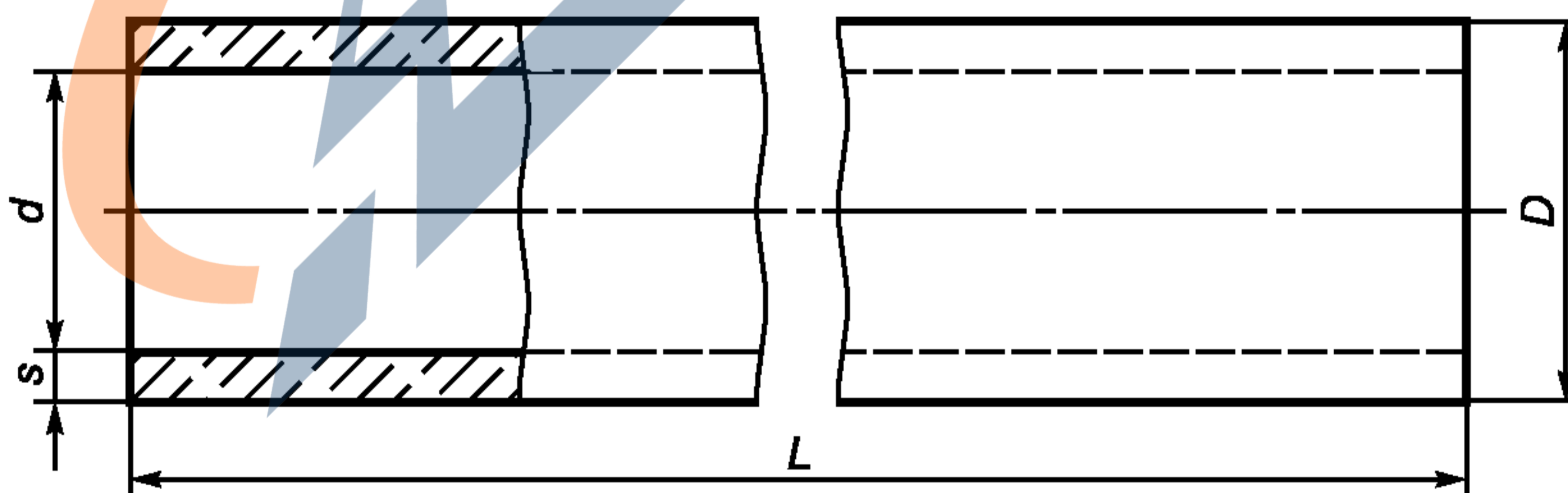
Рисунок 1 — Безнапорная труба
